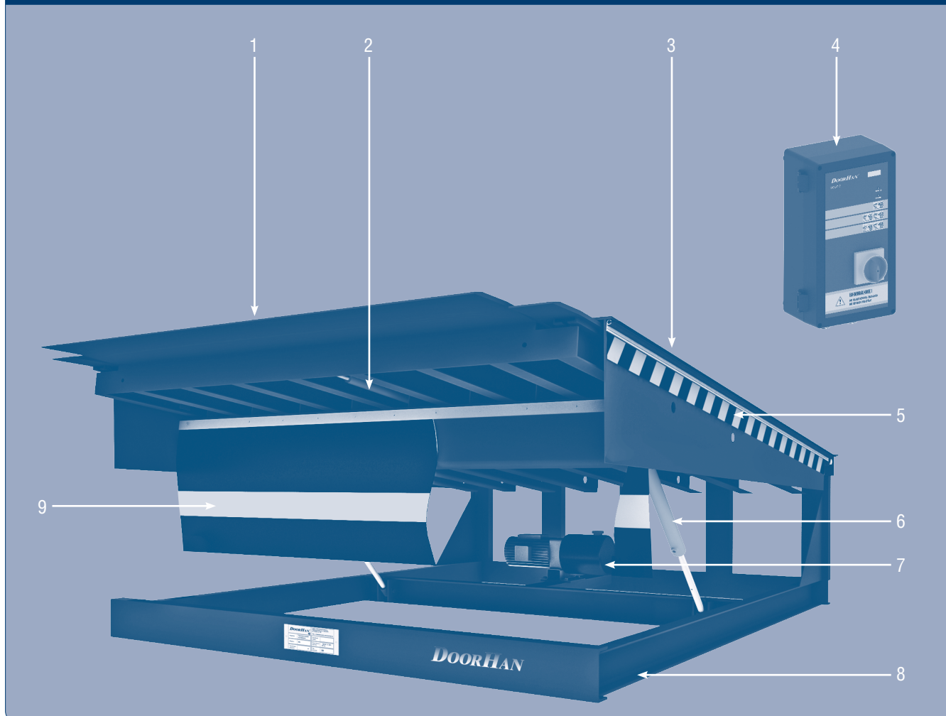
Рис. 4.1. Общий вид
